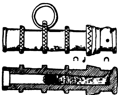
Abb. 282. Ansicht und Schnitt einer ungehäfteten Klotzbüchse aus Rom. Sammlung Forrer.
