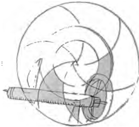
Abb. 833. Konstruktion eines Hebedaumens, 1438.
