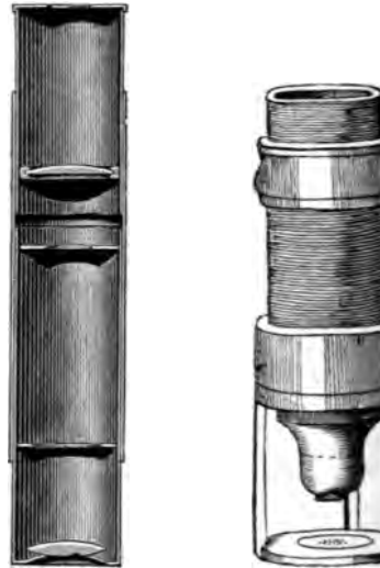
Abb. 475. Mikroskop, angeblich von Janssen. Abb. 476. Mikroskop von Campani.
