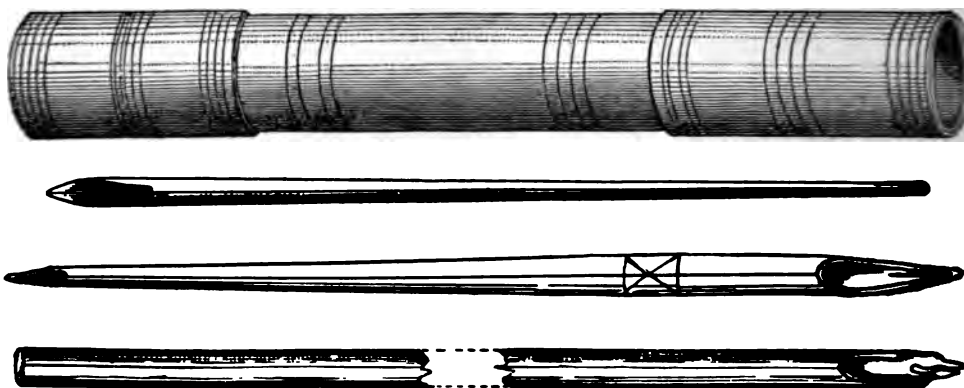
Abb. 662. Bronzene Büchse aus einem Römergrab von Frechen bei Köln, im Provinzial-Museum zu Bonn; dazu die obere Metallfeder und die Ziehfeder mit Rötelhalter Abb. 339. gehörig. Die mittlere Metallfeder stammt aus Avenches, aus dem 1. Jahrh. n. Chr.. Die unterste Metallfeder befindet sich im Museum zu Lüttich; sie wurde bei Tongres gefunden.
