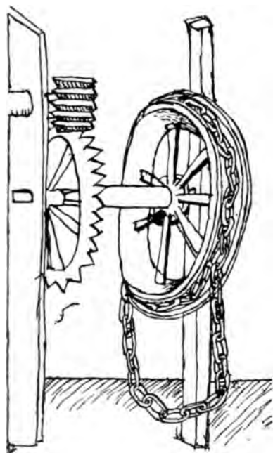
Abb. 379. Kettenantrieb nach Mariano, 1438.
