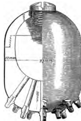
Abb. 361. Orsinibombe, 1858.
