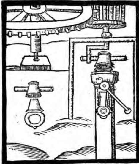
Abb. 334. Einschleifen der Hahnen, 1629, nach Branca.
