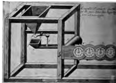
Abb. 567. Regenwaage von Leopold, 1726.
