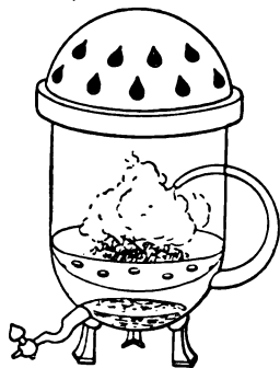
Abb. 124. Dampfgebläse nach Philon (Ausgabe von Carra de Vaux).
