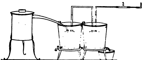
Abb. 234. Thermolampe. Nach C. Büniger, Die Thermolampe , Pirna 1802.
