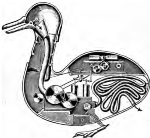
Abb. 30. Schnitt durch die Ente von Vaucanson.
