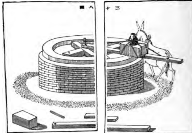
Abb. 626. Schleifen eines astronomischen Teilkreises nach Angabe der Jesuiten in China, um 1670. Holzschnitte aus der chinesischen Encyclopädie von 1726.
