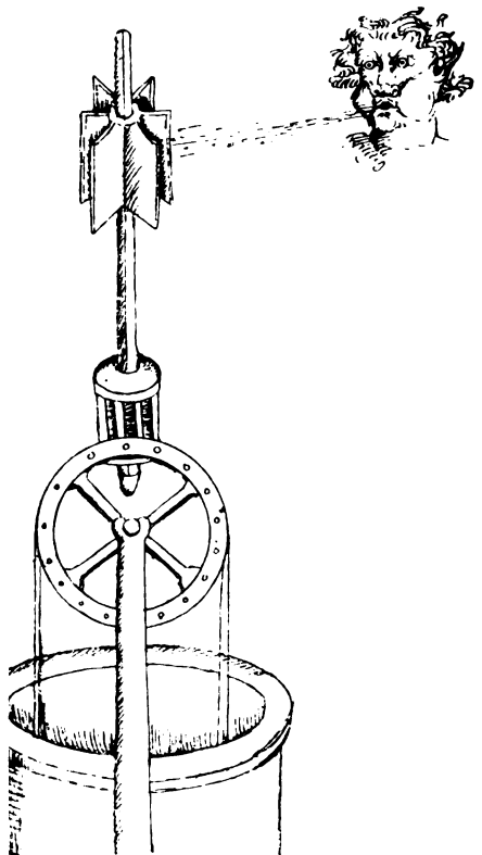
Abb. 811. Windturbine an einem Ziehbrunnen, nach Mariano, 1438.
