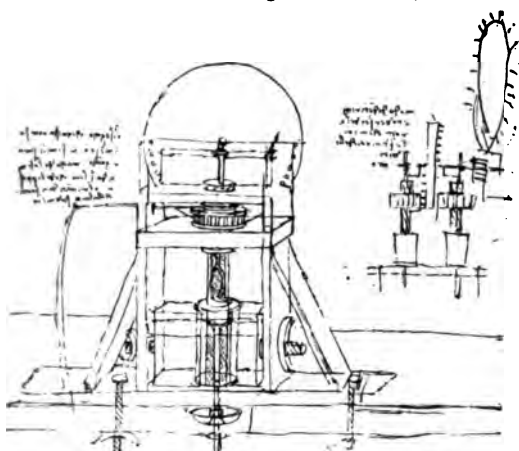
Abb. 624. Zylinder-Schleifmaschine, nach Leonardo da Vinci, um 1500.
