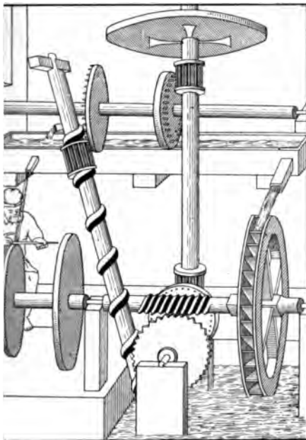
508. Perpetuum mobile nach der Strada- mandschrift um 1580; Kgl. Bibl. Berlin.
