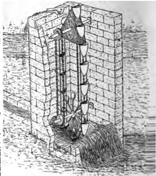
Abb. 542. Schöpfeimerkette nach Philon, um 230 v. Chr.
