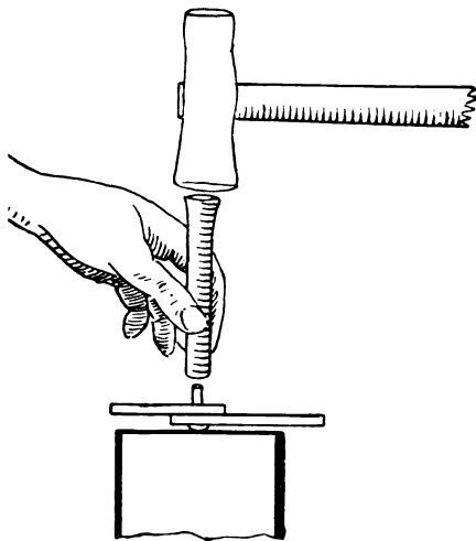
Abb. 495. Die Benutzung des Nietziehers.
