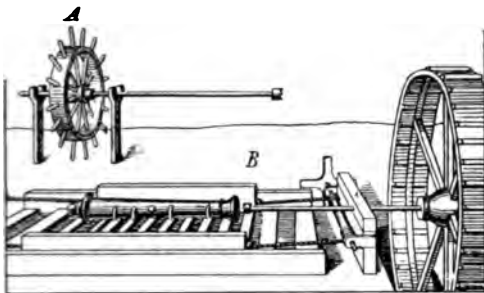
Abb. 258. Geschützbohrmaschine, 1540.
