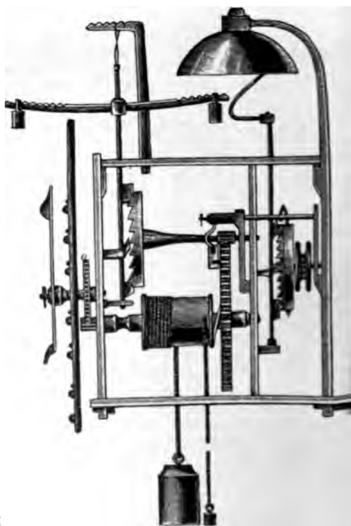
Abb. 775. Türmeruhr, um 1392, im Germanischen Museum Nürnberg. Nach Speckhart.
