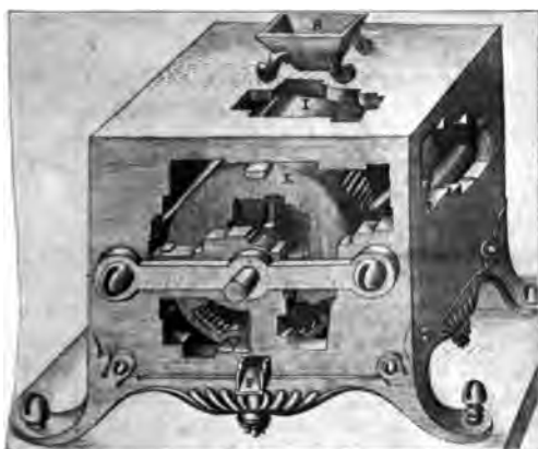
Abb. 484. Walzenmühle nach Ramelli, 1588.
