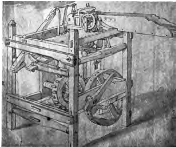
Abb. 328. Häcksellade mit automatischer Fortbewegung, Handzeichnung von 1695.
