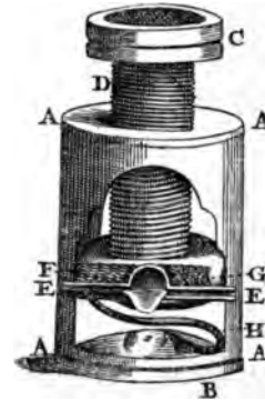
Abb. 458. Lupe von Wilson, 1700.
