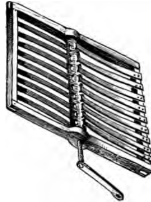
Abb. 227. Große Schnarre der Pfarrkirche zu Habelschwerdt.
