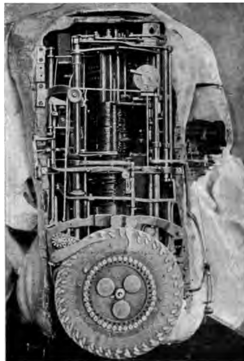
Abb. 33. Mechanismus des Schreibers. In der Mitte sieht man die Kurvenscheiben, unten die Einstellscheibe für das zu Schreibende.
