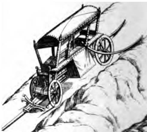
Abb. 357. Hemmstöcke unter den Hinterradnaben, nach Veranzio, 1595.
