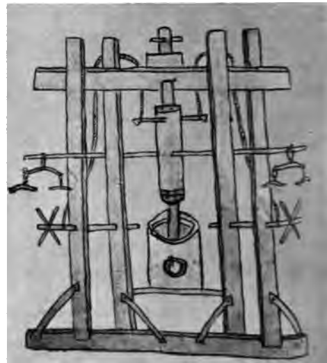
Abb. 256. Bohrmaschine für Geschütz, durch Göpel bewegt, um 1450.
